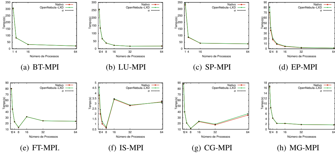
Figura 1. Resultados das aplicações da suíte NPB-MPI.
